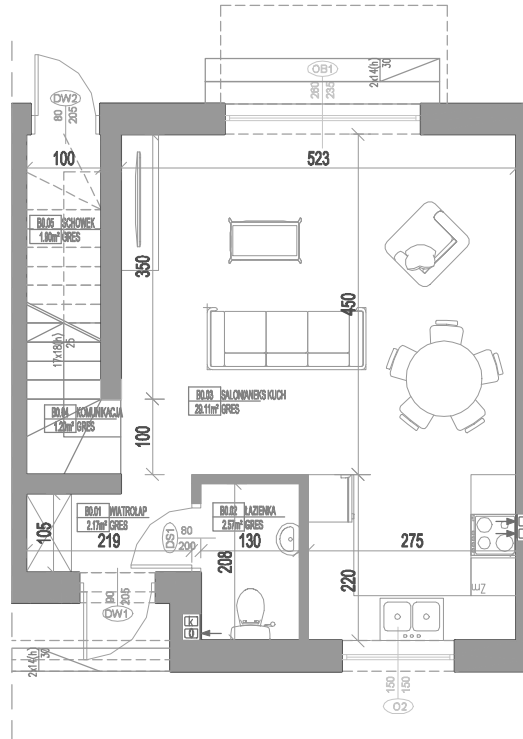
RZUT PARTERU LOKAL B
