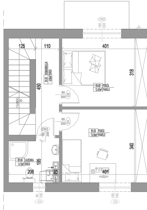
RZUT PIĘTRA LOKAL B
