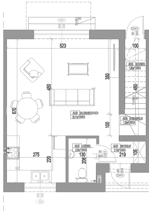
RZUT PARTERU LOKAL A
