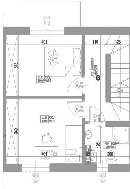
RZUT PIĘTRA LOKAL A
