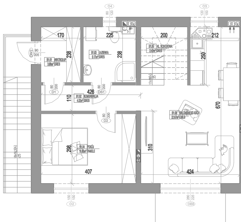
RZUT PIĘTRA LOKAL B
