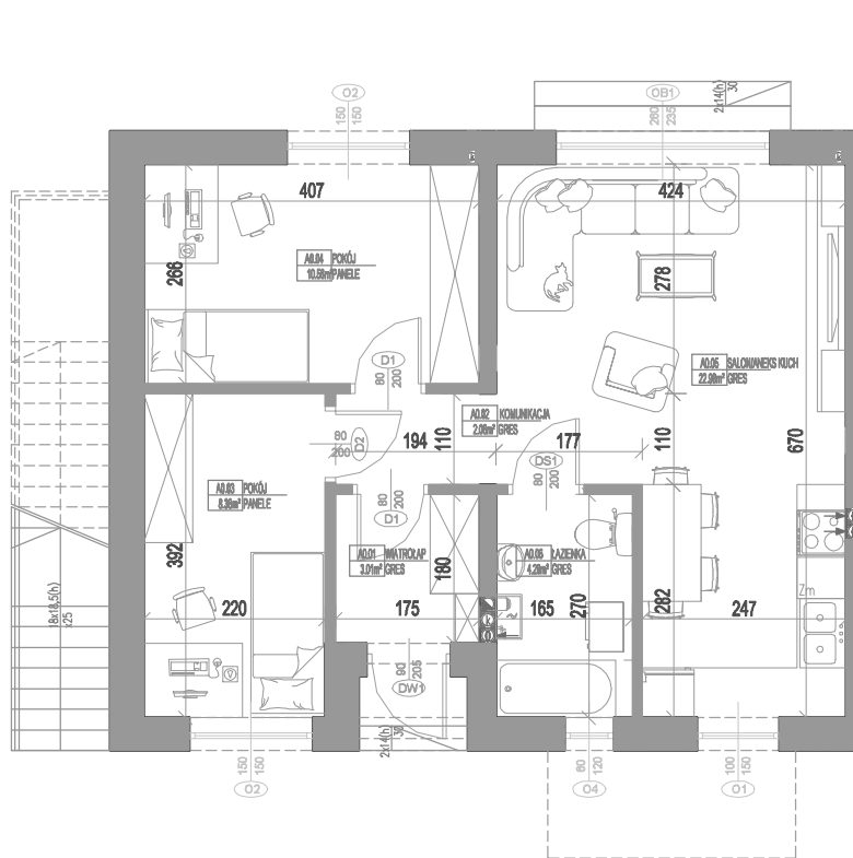
RZUT PARTERU LOKAL A
